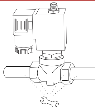
Oefen alleen kracht uit op aangegeven punten, nooit op de spoel of armatuur.
