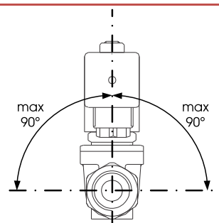
Maximale hoek 90°.
